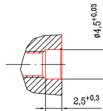
A-A (4:1)
