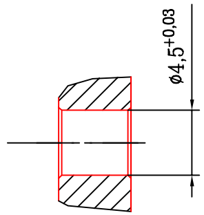
B-B (4:1)
