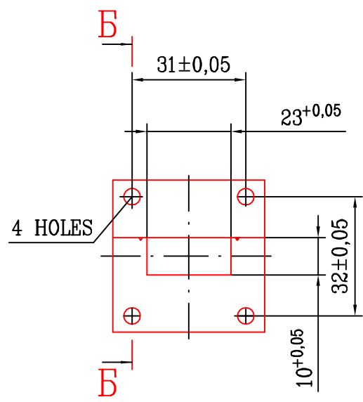
B-B (4:1)
